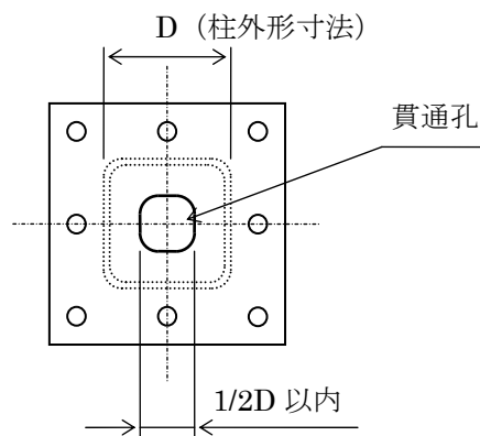
付図-1 ベースプレートの貫通孔
